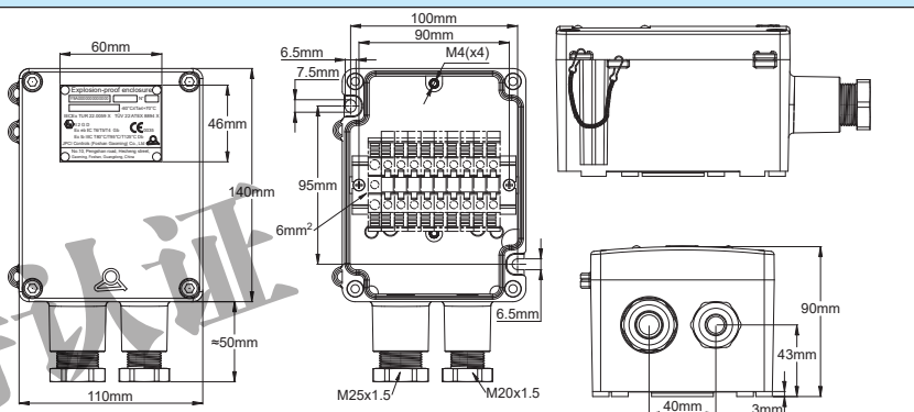
带接线柱的示例
